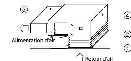
Retour d'air vers le bas (a)
